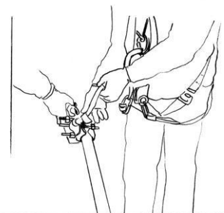
Preparazione punto d'ancoraggio
