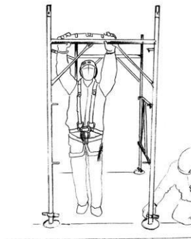
Regolazione trasversale telai
